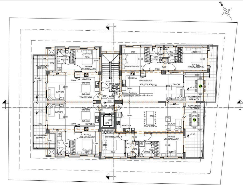
ΚΑΤΟΨΗ 1 ο ΟΡΟΦΟΥ
