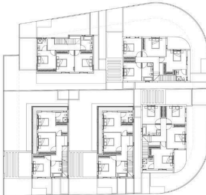
ΟΙΚΟΠΕΔΟ 3 - ΟΡΟΦΟΣ
