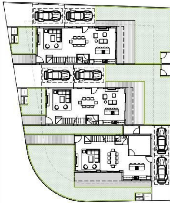
ΟΙΚΟΠΕΔΟ 1 - ΙΣΟΓΕΙΟ
