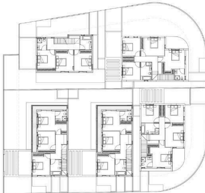
ΟΙΚΟΠΕΔΟ 3 - ΟΡΟΦΟΣ
