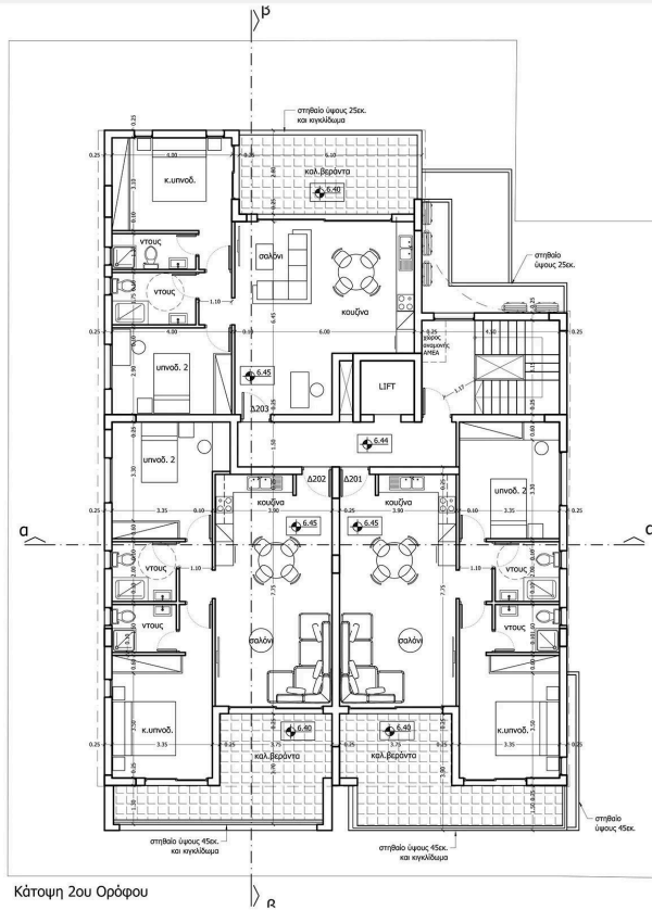
Κάτοψη 2ου Ορόφου
