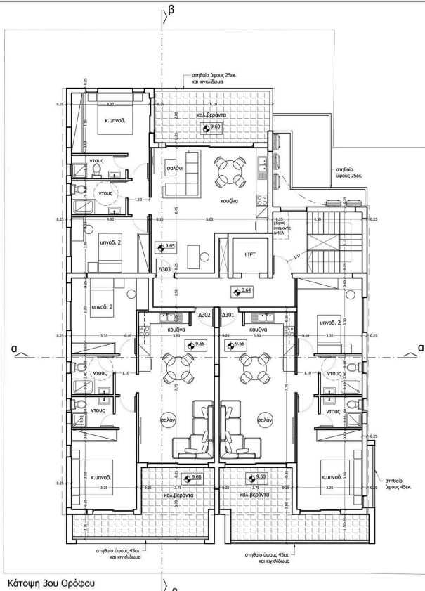
Κάτοψη 3ου Ορόφου
