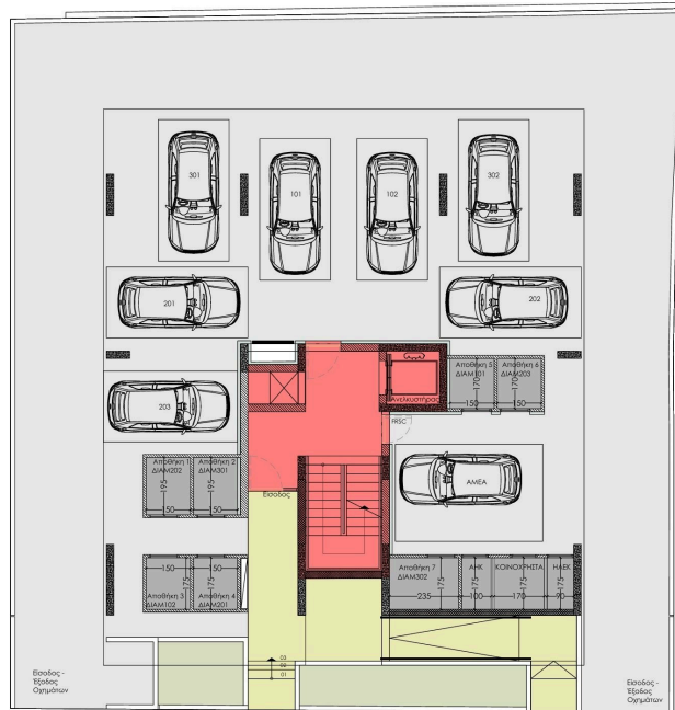
Κάτοψη ισογείου
