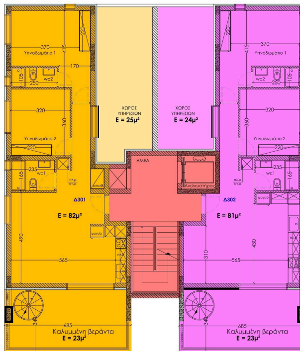
Κάτοψη 3ου ορόφου
