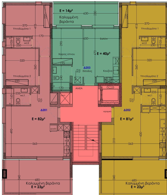
Κάτοψη 2ου ορόφου
