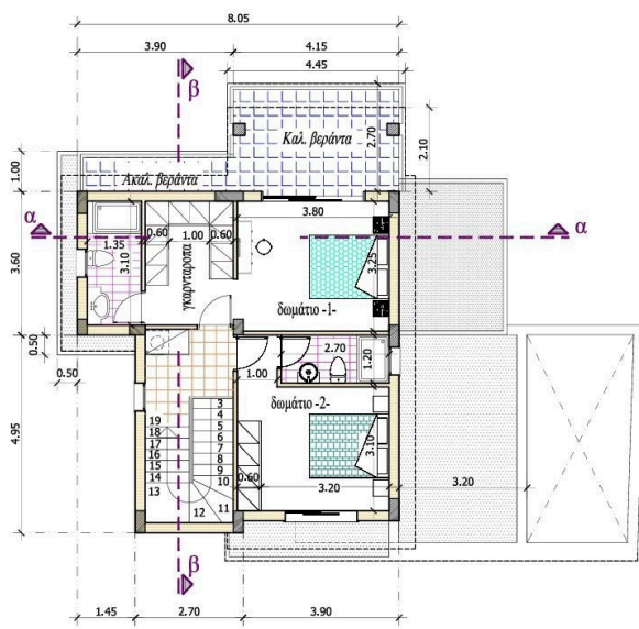
Κάτοψη α' ορόφου.
