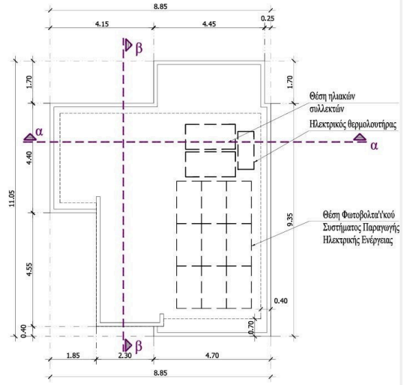
Κάτοψη ταράτσας.
