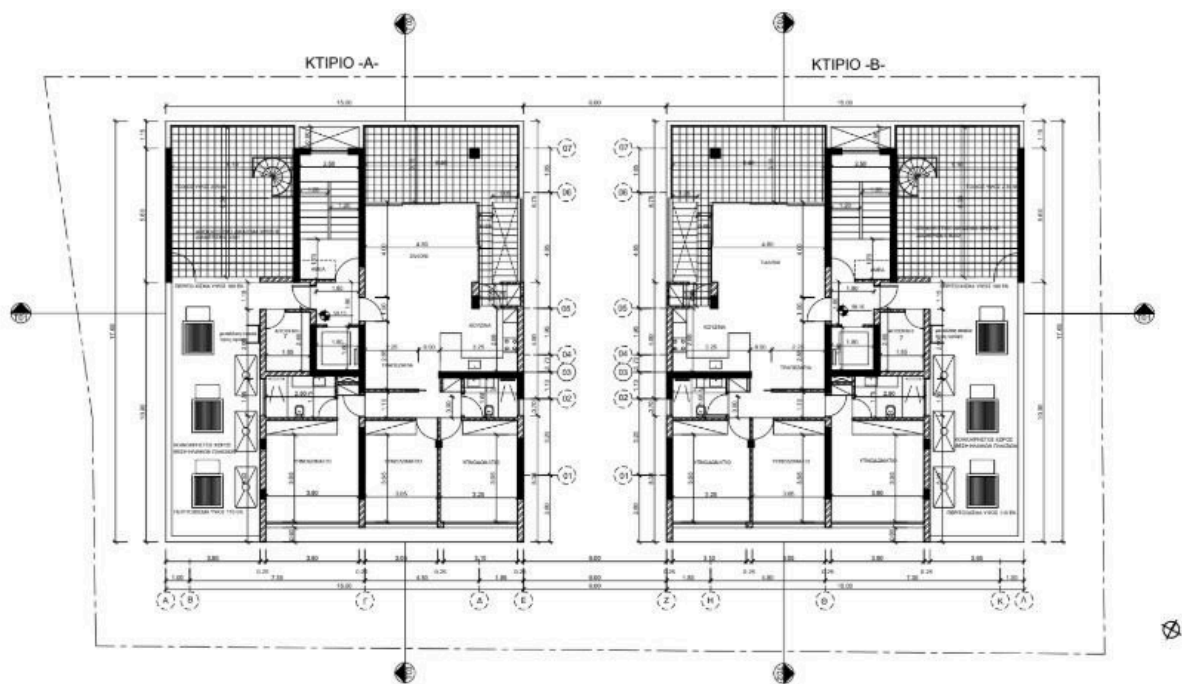
ΚΑΤΟΨΗ ΤΕΤΑΡΤΟΥ ΟΡΟΦΟΥ
