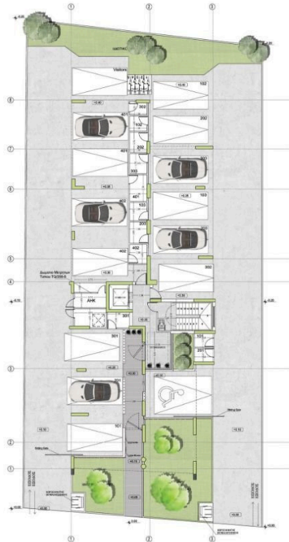
ΚΑΤΟΨΗ ΙΣΟΓΕΙΟΥ
