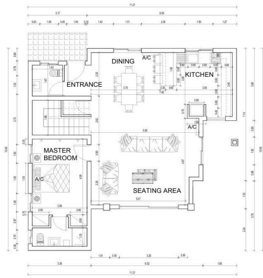
ΚΑΤΩΦΗ ΙΣΟΓΕΙΟΥ
