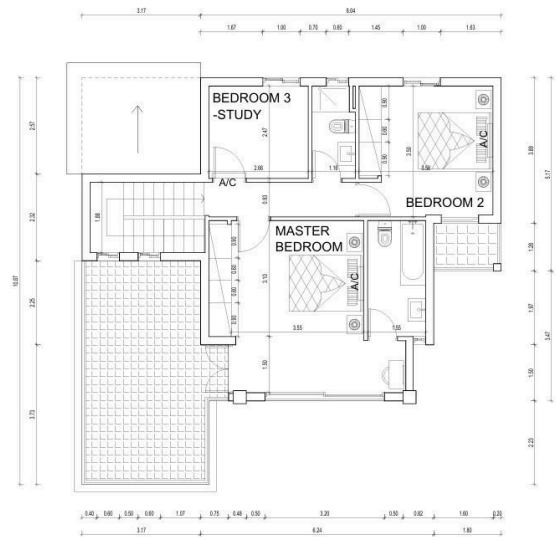
ΚΑΤΩΦΗ ΟΡΟΦΟΥ
