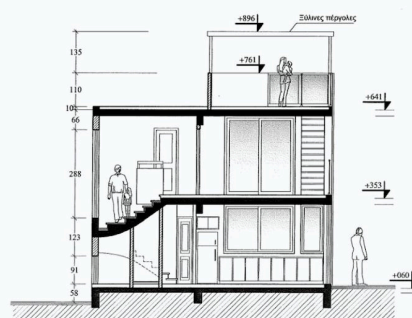
Τομή Α-Α
