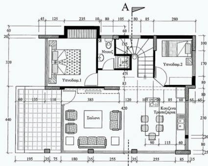
Κατοψη Ισογειου
