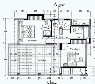
Κατοψη Οροφού
