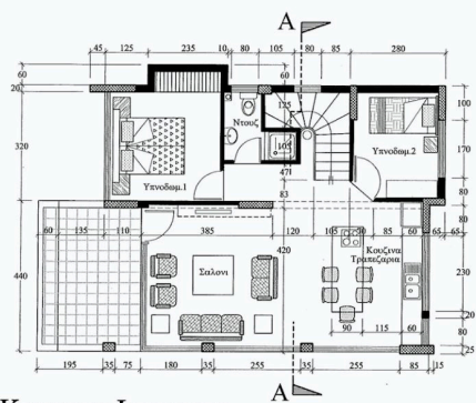
Κατοψη Ισογείου
