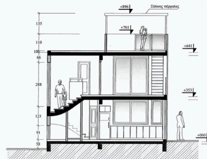
Τομή Α-Α
