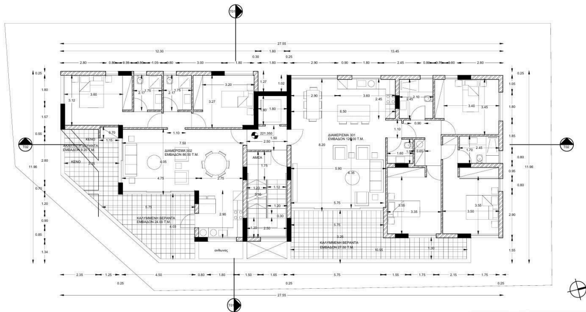
ΚΑΤΟΨΗ 3ΟΥ ΟΡΟΦΟΥ
