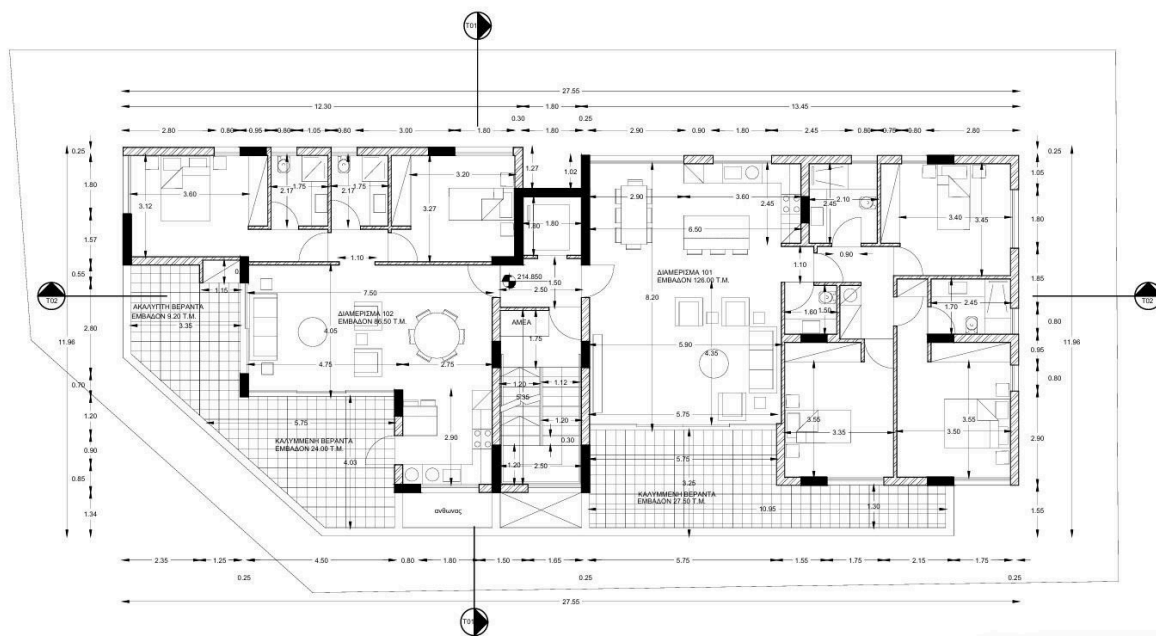
ΚΑΤΟΨΗ 1ΟΥ ΟΡΟΦΟΥ
