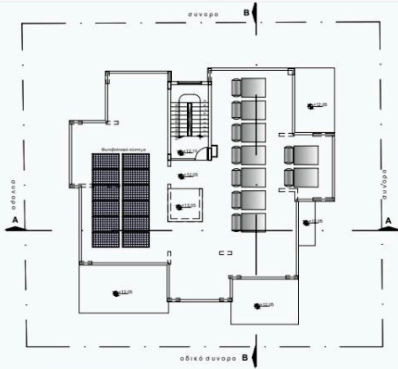
ΚΑΤΟΨΗ ΟΡΟΦΗΣ ΚΛΙΜΑΚΑ 1:200
