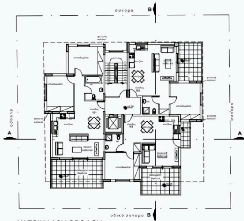
ΚΑΤΟΨΗ 3ΟΥ ΟΡΟΦΟΥ ΚΛΙΜΑΚΑ 1:200
