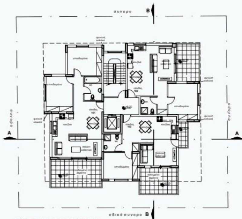
ΚΑΤΟΨΗ 2ΟΥ ΟΡΟΦΟΥ ΚΛΙΜΑΚΑ 1:200
