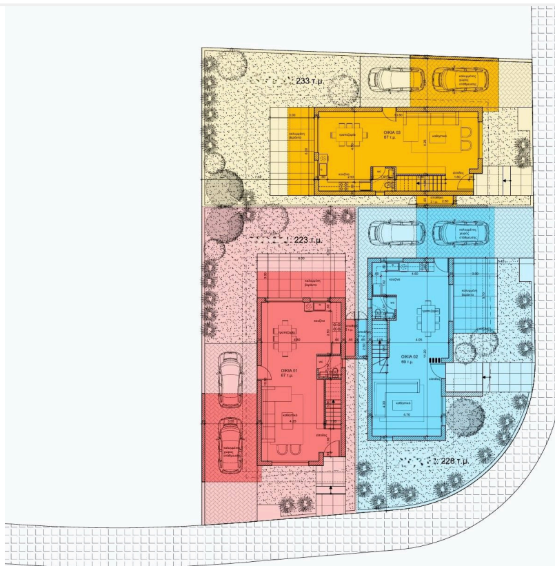
Ισόγειο
