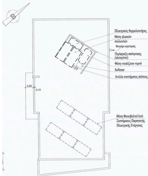
Κάτοψη ταρράτσας. κλ. 1:100
