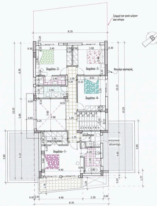
Κάτοψη 1ου ορόφου. κλ. 1:100
