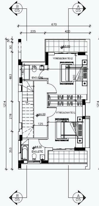
ΚΑΤΩΦΗ ΟΡΟΦΟΥ
