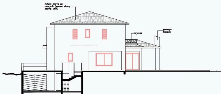
ΟΠΙΣΘΙΑ ΟΨΗ
