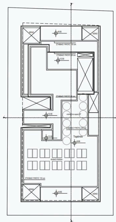
ΚΑΤΟΨΗ ΤΑΡΑΤΣΩΝ
