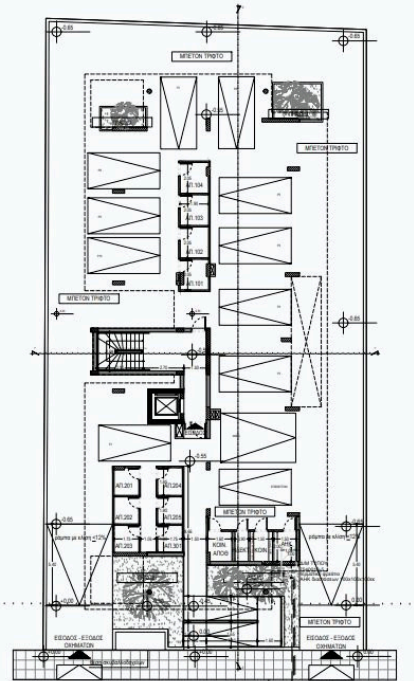
ΚΑΤΟΨΗ ΥΠΟΣΤΕΓΟΥ
