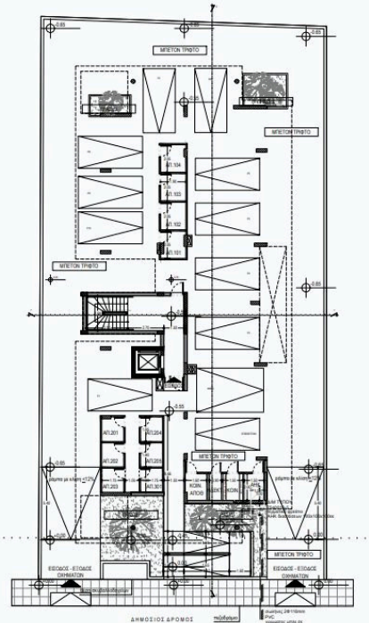
ΚΑΤΟΨΗ ΥΠΟΣΤΕΓΟΥ
