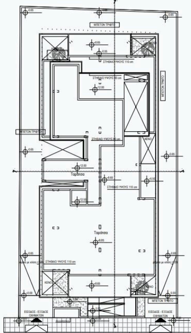
ΓΕΝΙΚΟ ΧΩΡΟΤΑΞΙΚΟ
