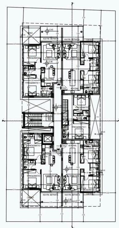
ΚΑΤΟΨΗ 1ου ΟΡΟΦΟΥ
