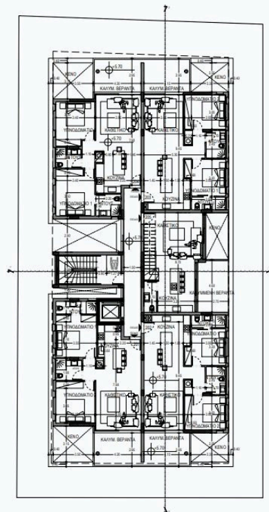
ΚΑΤΟΨΗ 2ου ΟΡΟΦΟΥ
