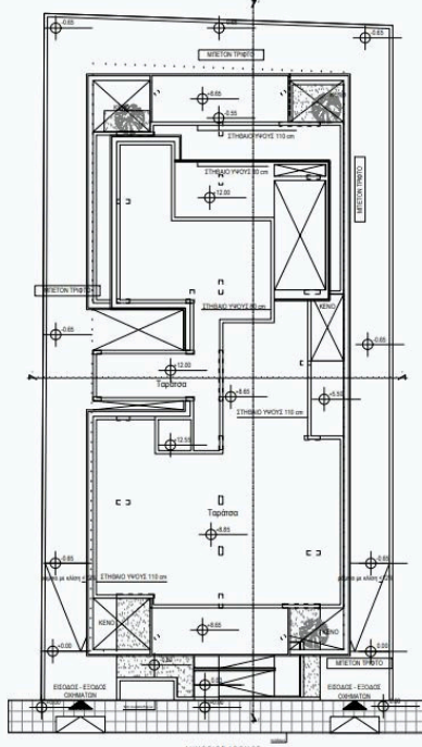
ΓΕΝΙΚΟ ΧΩΡΟΤΑΞΙΟ
