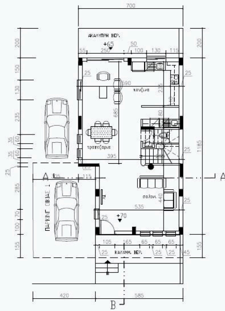
ΤΥΠΟΣ Α ΚΑΤΟΨΗ ΙΣΟΓΕΙΟΥ
