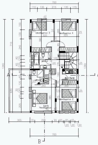
ΤΥΠΟΣ Α ΚΑΤΟΨΗ ΟΡΟΦΟΥ
