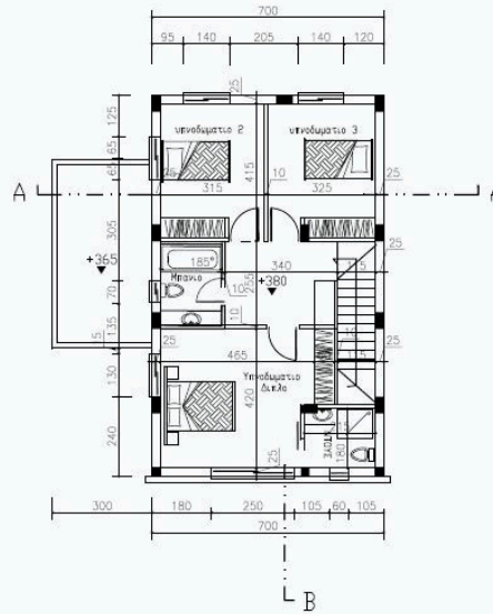
ΤΥΠΟΣ Β ΚΑΤΟΨΗ ΟΡΟΦΟΥ
