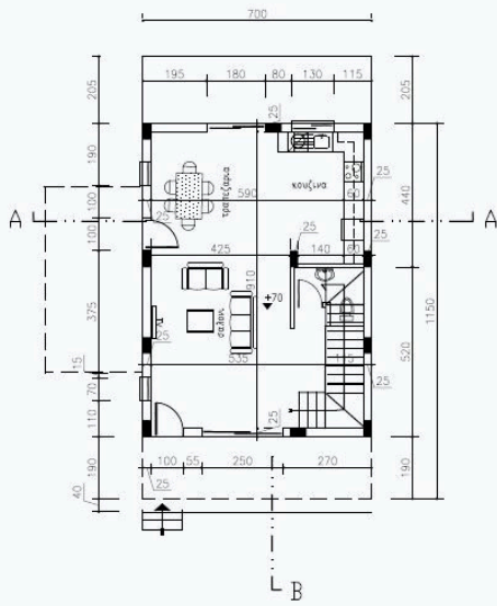
ΤΥΠΟΣ Β ΚΑΤΟΨΗ ΙΣΟΓΕΙΟΥ
