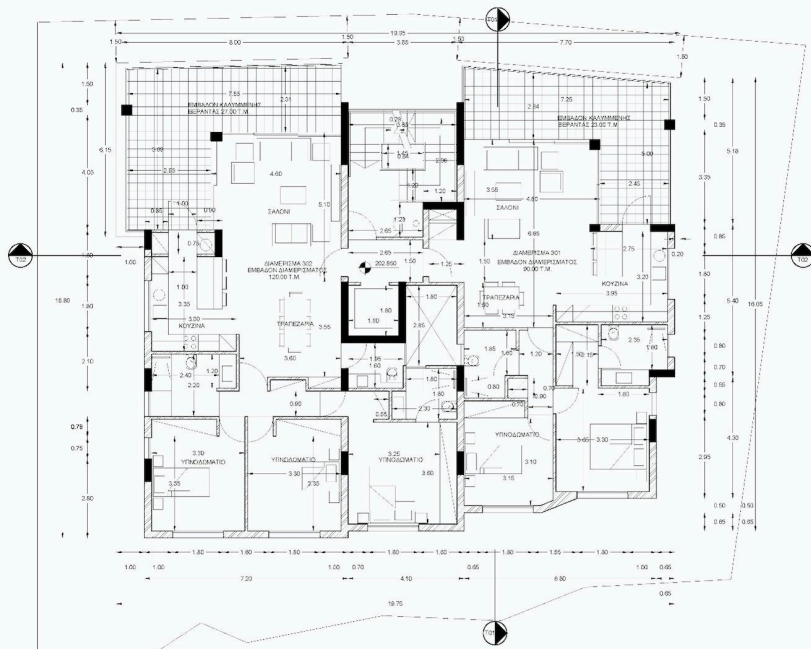
ΚΑΤΟΨΗ 3ΟΥ ΟΡΟΦΟΥ
