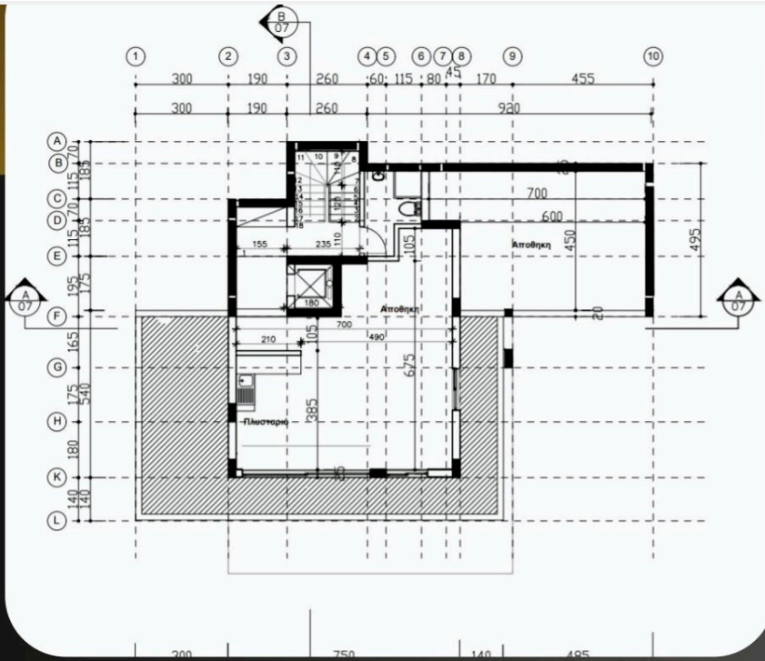
BASSEMENT FLOOR PLAN
