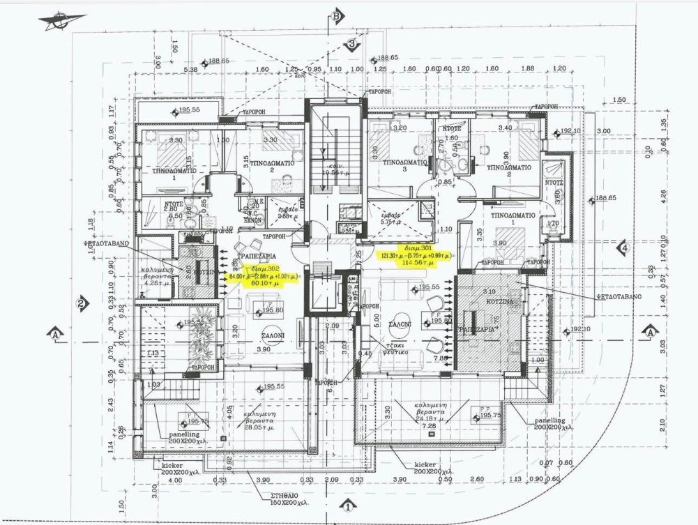
ΚΑΤΩΦΗ 3ου ΟΡΟΦΟΥ 230.19τ.μ. - (2.88τ.μ.+0.87τ.μ.+1.00τ.μ.+2.88τ.μ.+1.02τ.μ.+0.99τ.μ.+5.75τ.μ.+0.58τ.μ.)=214.22τ.μ.
