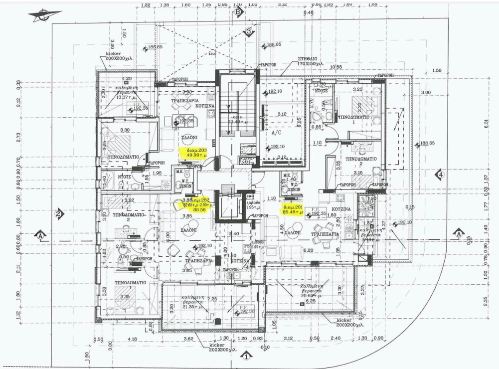
ΚΑΤΩΦΗ 2ου ΟΡΟΦΟΥ 248.60τ.μ. - (2.88τ.μ.+1.00τ.μ.+1.05τ.μ.+2.09τ.μ.+1.95τ.μ.+0.58τ.μ.)=239.05τ.μ.
