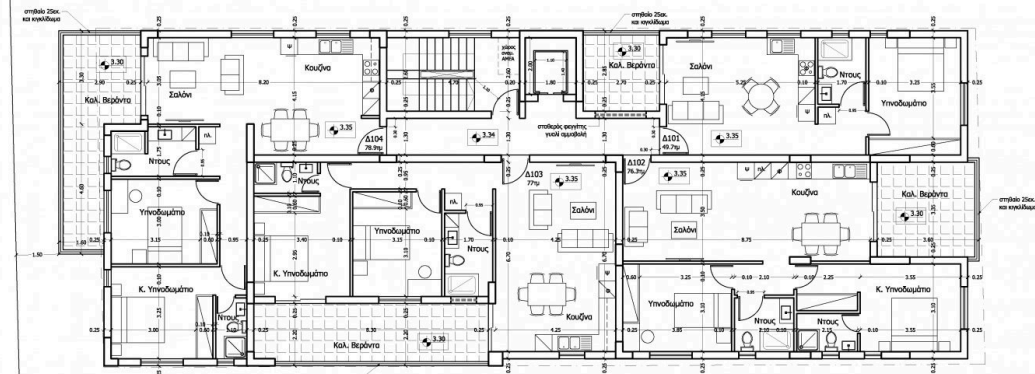
Κάτοψη 1ου Ορόφου
