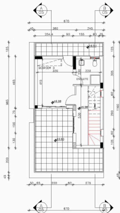
ΚΑΤΟΨΗ ΟΡΟΦΗΣ ΚΛΙΜΑΚΟΣΤΑΣΙΟΥ
