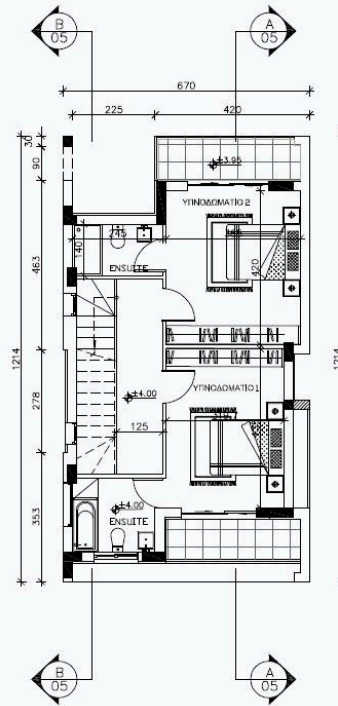
ΚΑΤΟΨΗ ΟΡΟΦΟΥ
