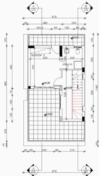
ΚΑΤΩΦΗ ΟΡΟΦΗΣ ΚΛΙΜΑΚΟΣΤΑΣΙΟΥ
