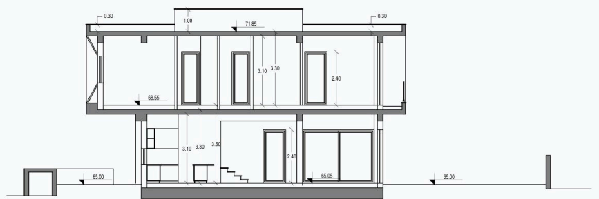
ΤΟΜΗ Β-Β' ΚΛΙΜΑΚΑ 1:100
