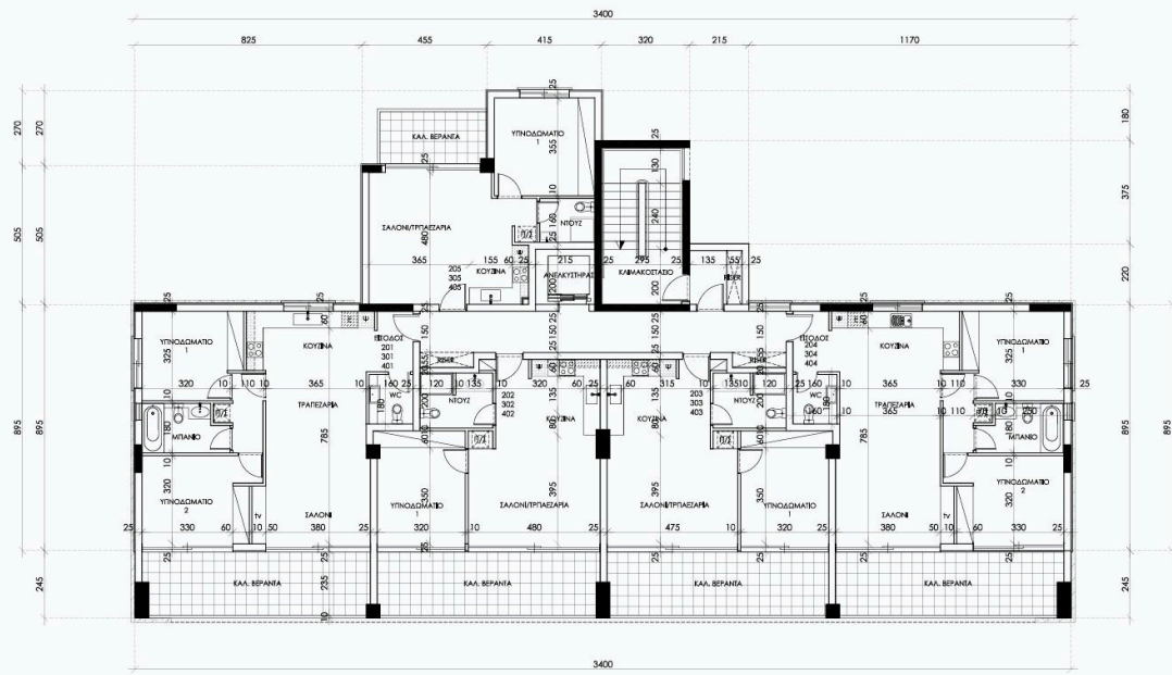
NEA ΚΑΤΟΨΗ ΤΥΠΙΚΟΥ ΟΡΟΦΟΥ (2ΟΙ-4ΟΙ ΟΡΟΦΟΙ)
