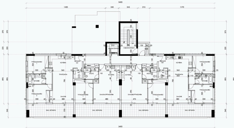
ΝΕΑ ΚΑΤΩΗ ΠΡΩΤΟΥ ΟΡΟΦΟΥ
