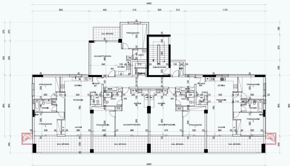
NEA ΚΑΤΟΨΗ ΠΕΜΠΤΟΥ ΟΡΟΦΟΥ
