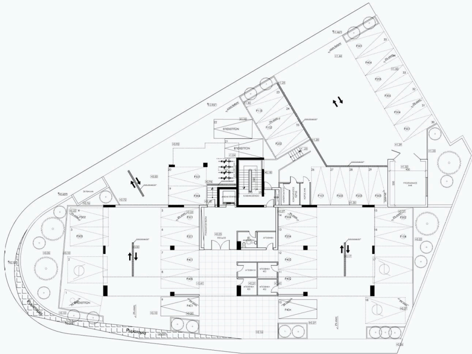
ΚΑΤΩΗ ΙΣΟΓΕΙΟΥ / ΧΩΡΟΣΑΙΚΟ
