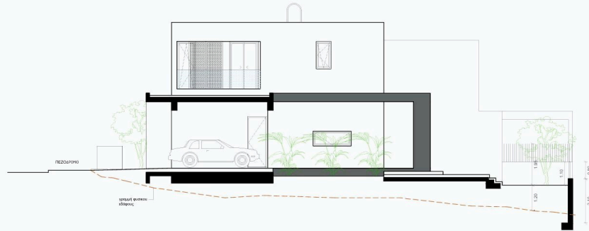
ΝΟΤΙΟΔΥΤΙΚΗ ΟΨΗ
