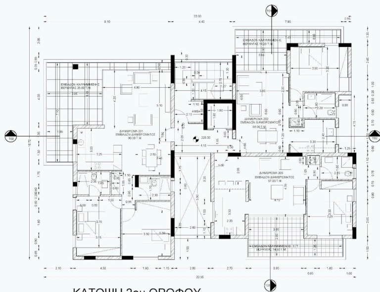
ΚΑΤΟΨΗ 2ου ΟΡΟΦΟΥ
