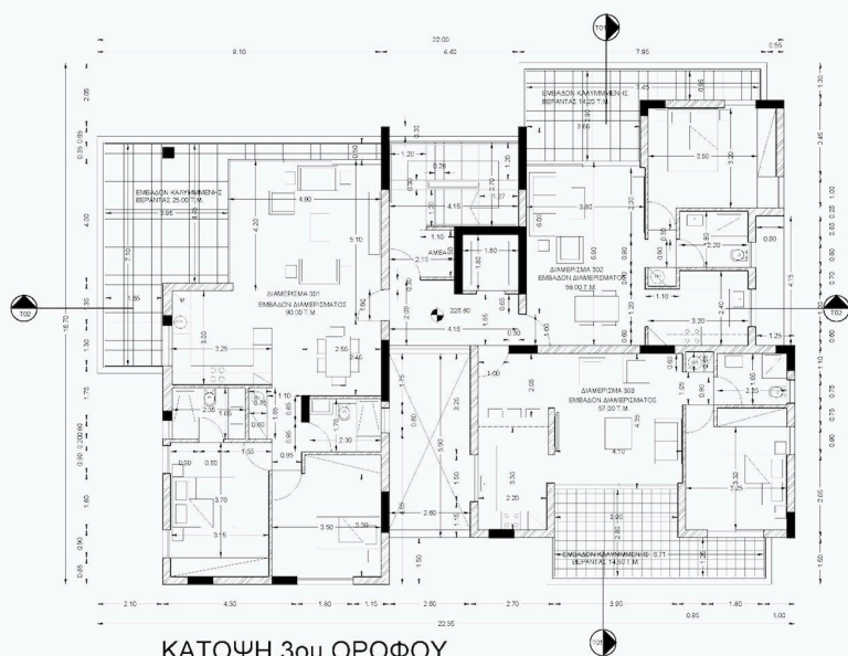
ΚΑΤΟΨΗ 3ου ΟΡΟΦΟΥ
