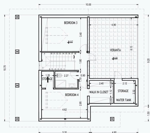
ΚΑΤΩΦΗ ΣΟΦΙΤΑΣ ΚΛΙΜΑΚΑ 1:100
