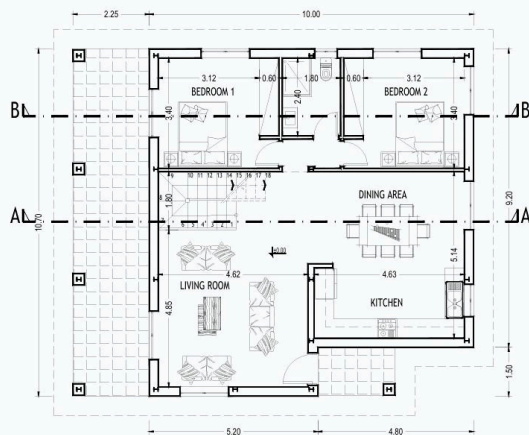
ΚΑΤΩΦΗ ΙΣΟΓΕΙΟΥ ΚΛΙΜΑΚΑ 1:100
