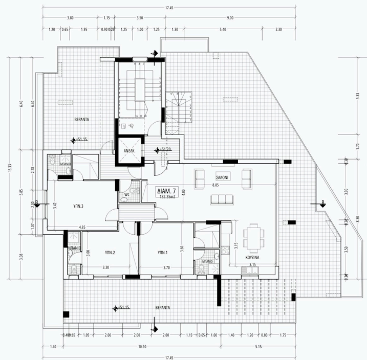
ΚΑΤΩΨΗ Γ' ΟΡΟΦΟΥ ΛΥΣΗ Δ'
