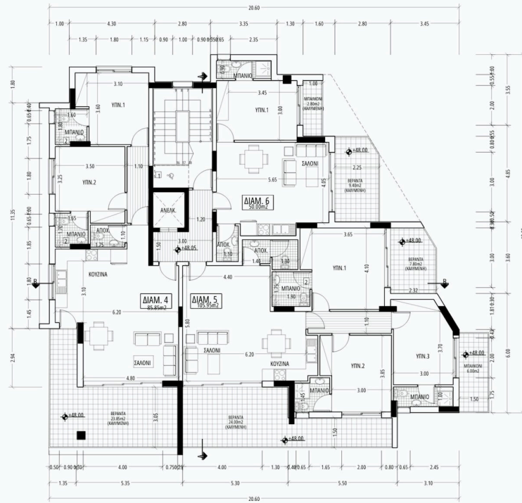
ΚΑΤΩΨΗ Β' ΟΡΟΦΟΥ
