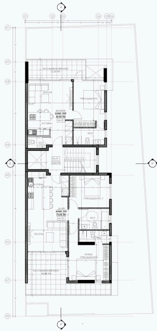
ΚΑΤΩΦΗ 2ΟΥ ΟΡΟΦΟΥ
