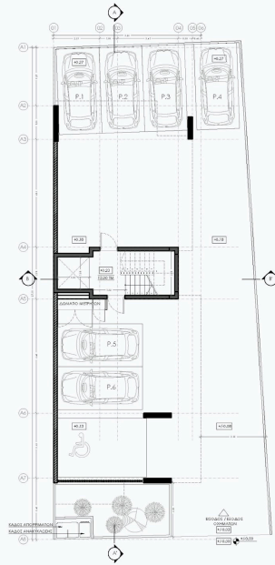
ΚΑΤΟΨΗ ΙΣΟΓΕΙΟΥ
