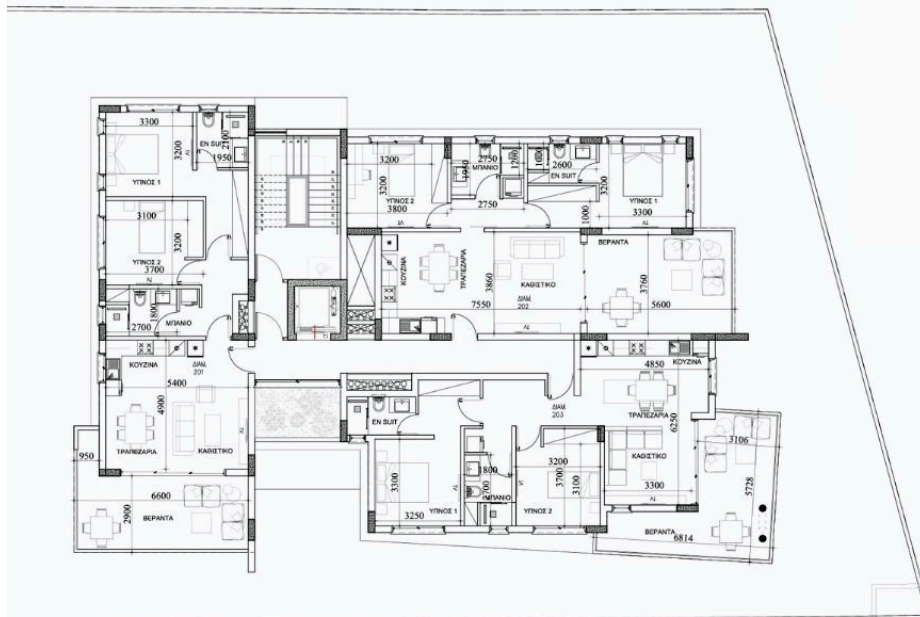
ΚΑΤΩΦΗ 2ου ΟΡΟΦΟΥ ΚΥΜΑΝΣΑ 1:100
