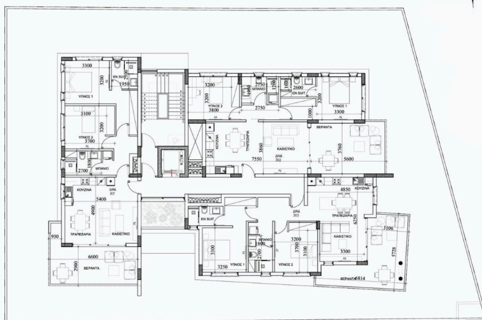
ΚΑΤΩΦΗ 3ου ΟΡΟΦΟΥ ΚΥΜΑΝΣΑ 1:100
