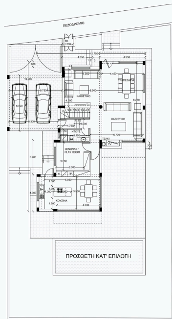
ΚΑΤΟΨΗ ΙΣΟΓΕΙΟΥ
