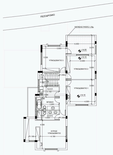
ΚΑΤΟΨΗ ΟΡΟΦΟΥ
