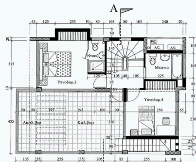
Κατοψη Οροφου
