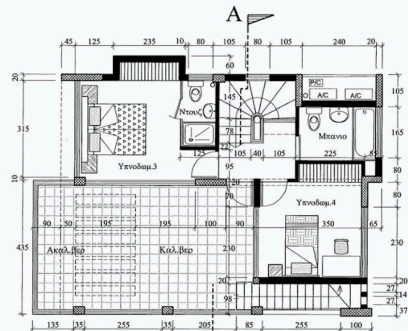
Κατοψη Οροφου
