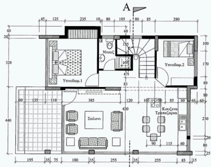
Κατοψη Ισογείου
