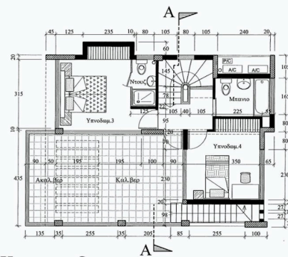
Κατοψη Οροφού
