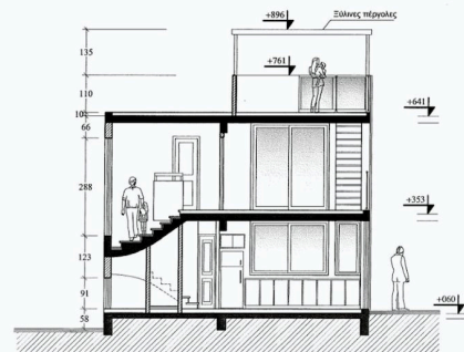
Τομη Α-Α
