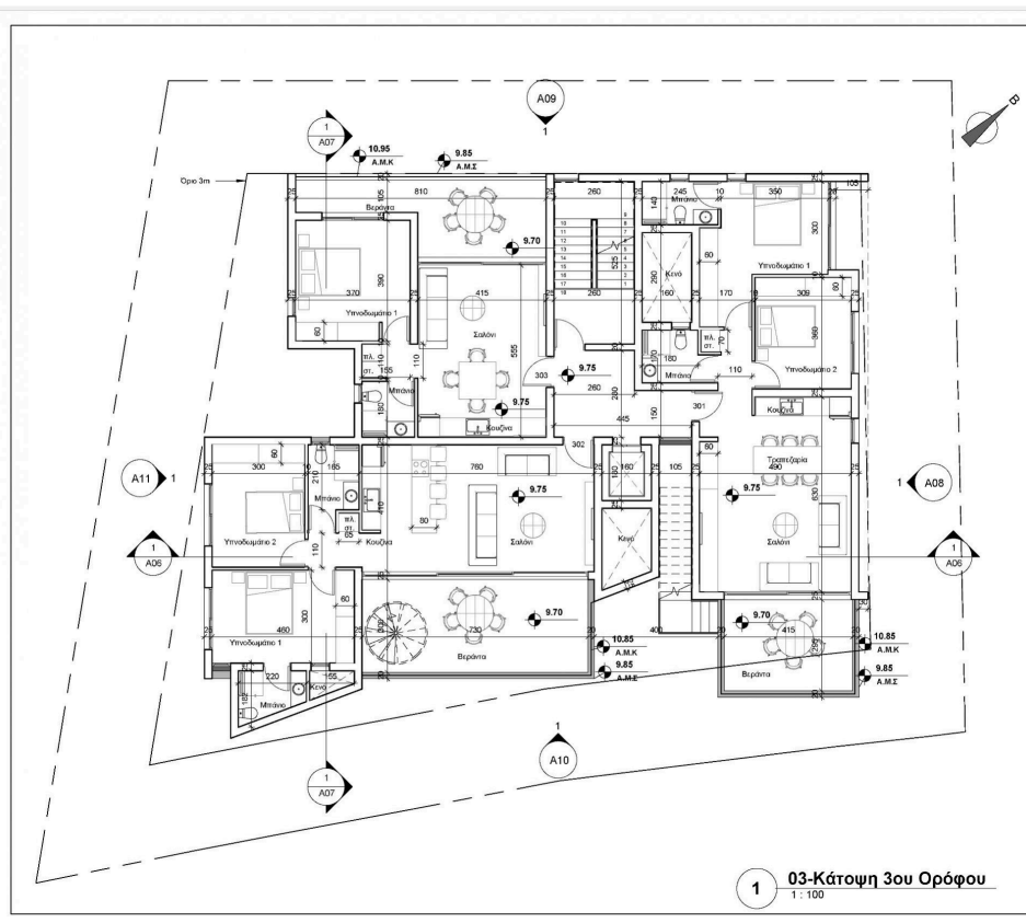
1 02 - Κάτοψη 2ου Ορόφου 1 : 100
