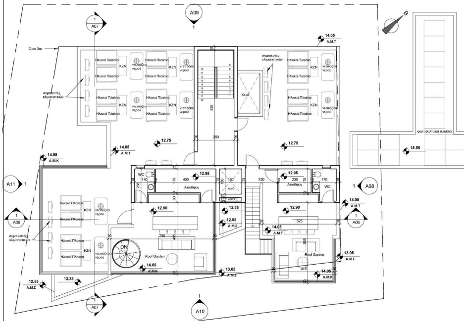
1 04-Κάτοψη Οροφής 1 : 100
