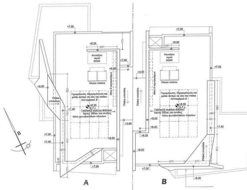
ΚΑΤΩΦΗ ΟΡΟΦΗΣ ΚΑ. 1:100
