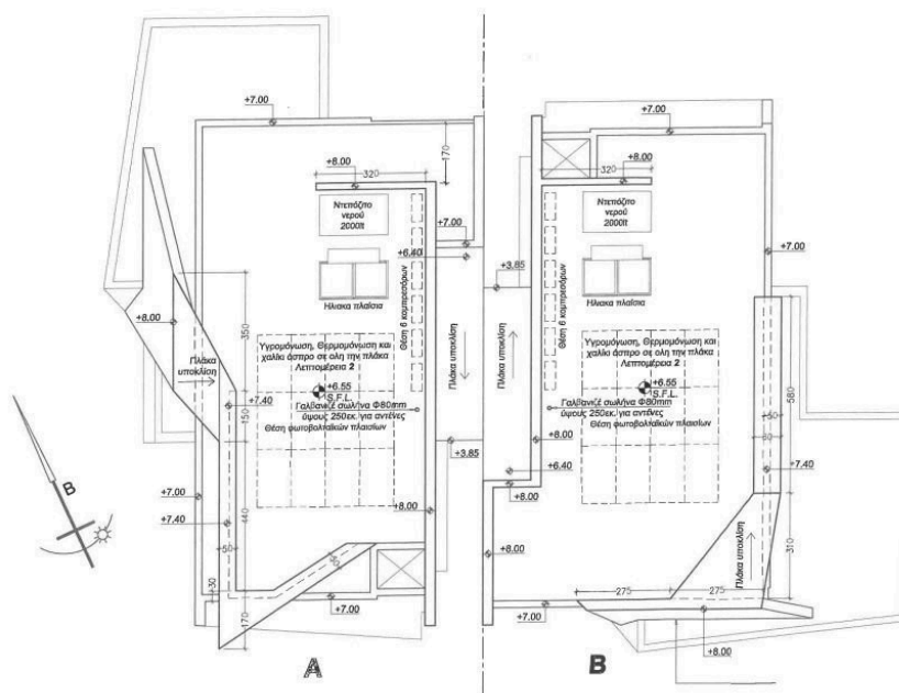
ΚΑΤΩΦΗ ΟΡΟΦΗΣ ΚΑ. 1:100
