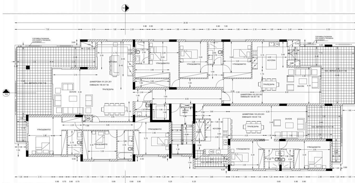
ΚΑΤΟΨΗ ΤΥΠΙΚΟΥ ΟΡΟΦΟΥ
