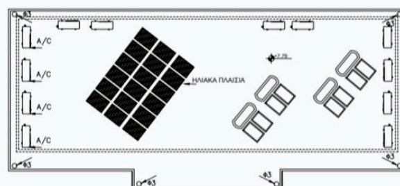
ΚΑΤΟΨΗ ΟΡΟΦΗΣ
