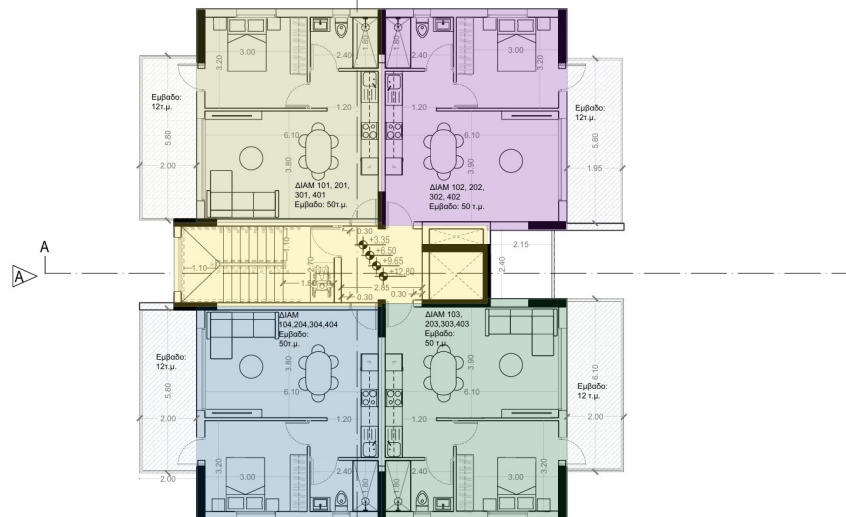
ΚΑΤΟΨΗ 1ΟΥ- 4ΟΥ ΟΡΟΦΟΥ
