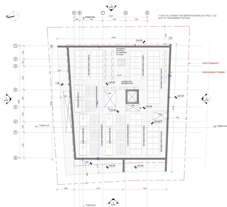
A004-ΕΠΙΠΕΔΟ ΟΡΟΦΗΣ 1 : 100
