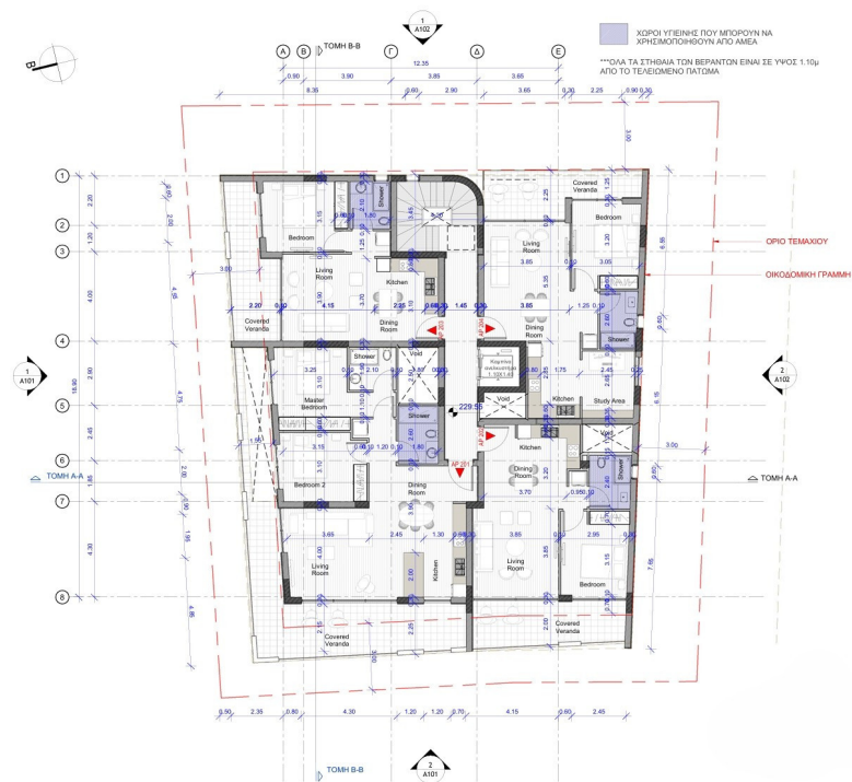
A003-ΕΠΙΠΕΔΟ 2ου ΟΡΟΦΟΥ 1 : 100
