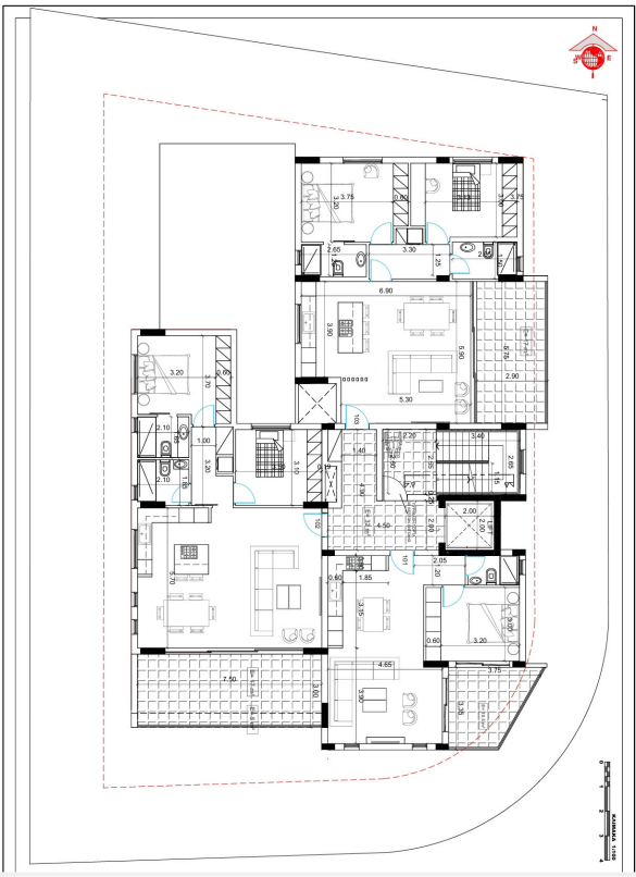
ΚΑΤΟΨΗ 1ου ΟΡΟΦΟΥ
