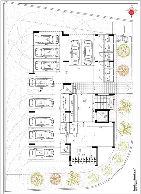
ΚΑΤΟΨΗ ΙΣΟΓΕΙΟΥ
