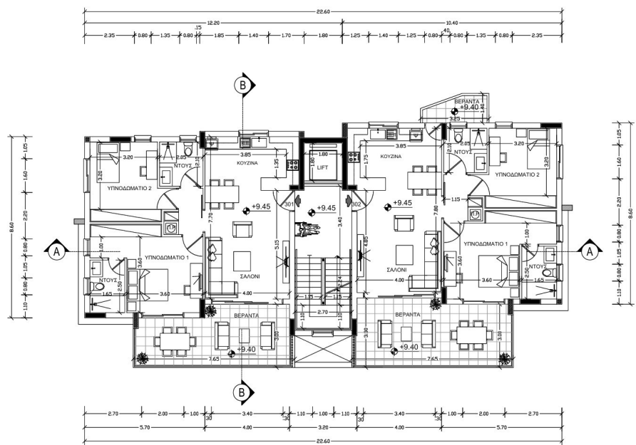
ΚΑΤΟΨΗ 3ου ΟΡΟΦΟΥ ΚΛΙΜΑΚΑ 1:100
