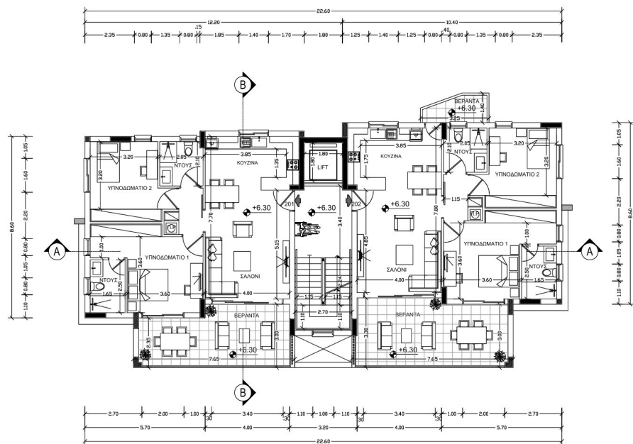
ΚΑΤΟΨΗ 2ου ΟΡΟΦΟΥ ΚΛΙΜΑΚΑ 1:100
