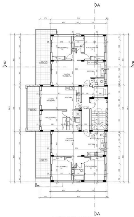
ΚΑΤΩΗ ΤΡΙΤΟΥ ΟΡΟΦΟΥ BLOCK E
