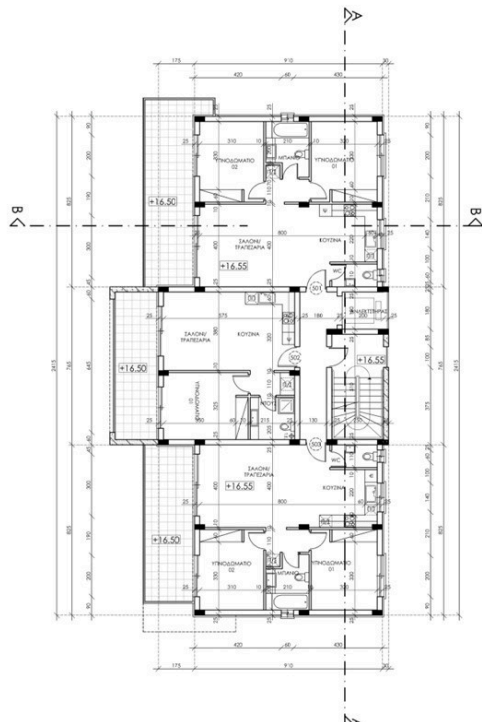
ΚΑΤΟΠΗ ΠΕΜΠΤΟΥ ΟΡΟΦΟΥ BLOCK E
