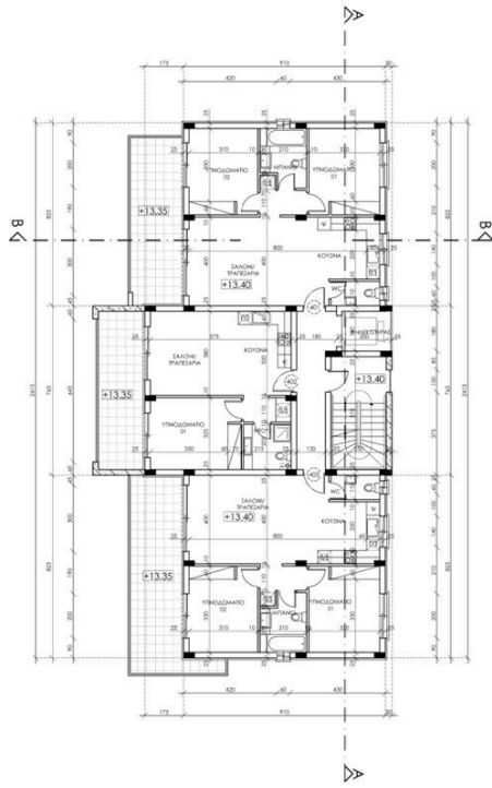
ΚΑΤΟΠΗ ΤΕΤΑΡΤΟΥ ΟΡΟΦΟΥ BLOCK E
