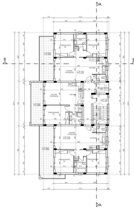
ΚΑΤΩΗ ΔΕΥΤΕΡΟΥ ΟΡΟΦΟΥ BLOCK E
