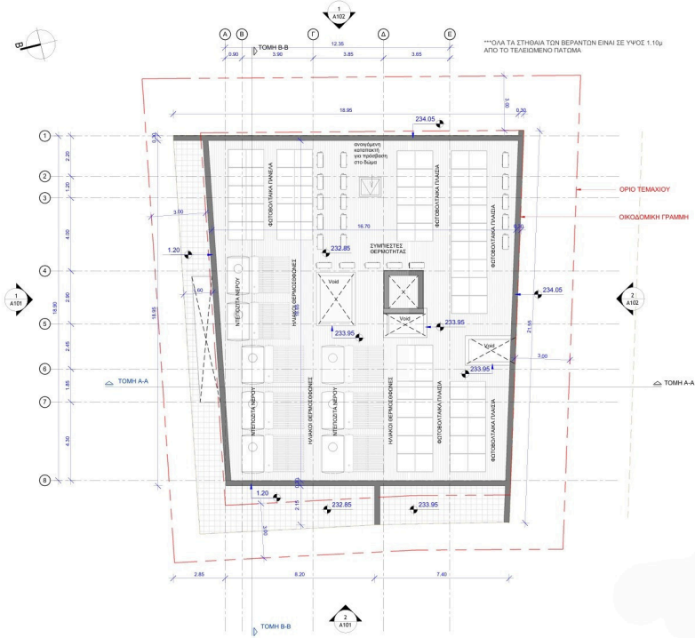
A004-ΕΠΙΠΕΔΟ ΟΡΟΦΗΣ 1 : 100
