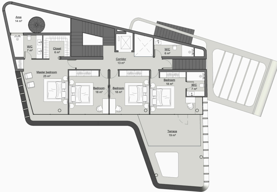
1 B1 Level 3 1 : 100
